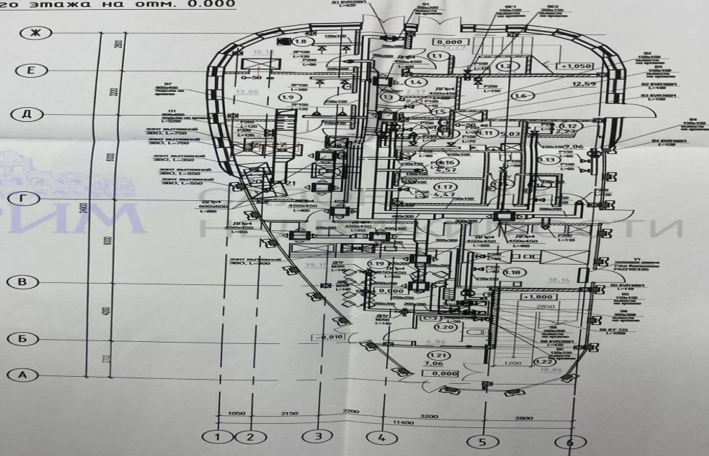
План 1-20 этажа на отм. 0.000
